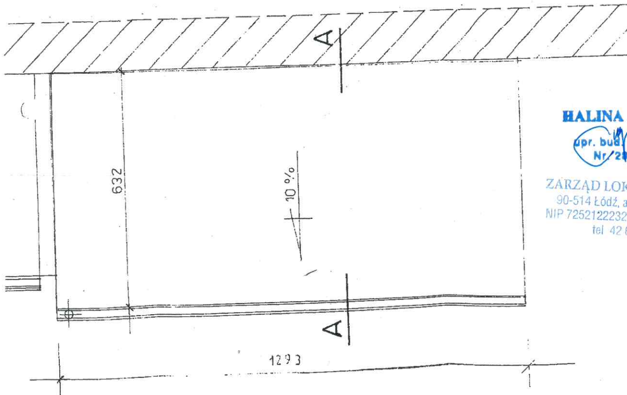
Rzut dachu 1:100
