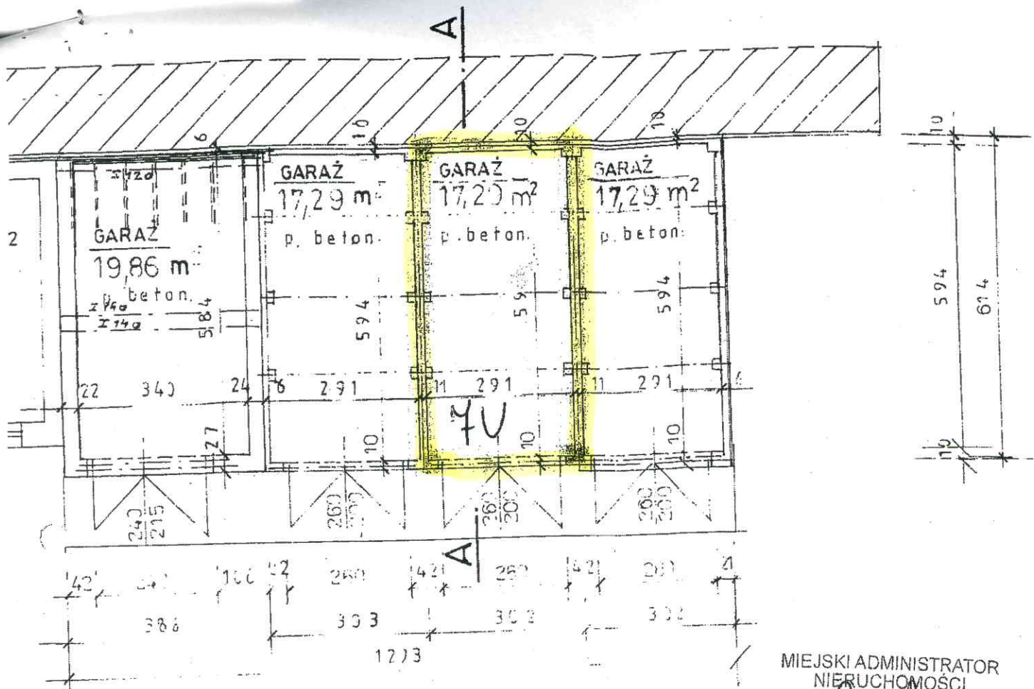
Rzut przyziemia 1:100
